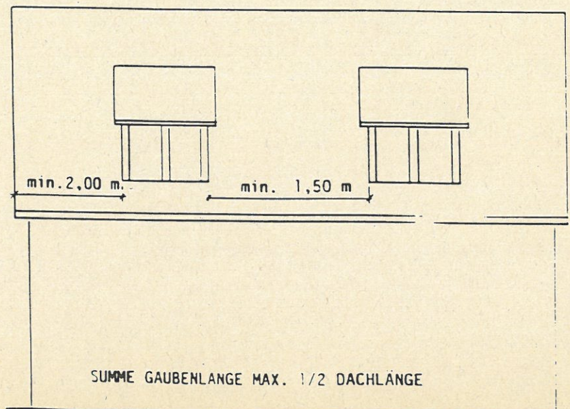
SCHLEPPGAUBEN
